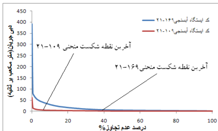
شکل ۲: منحنی تداوم جریان دو حوزه با مشخصات هندسی و هیدرولوژیکی مختلف
